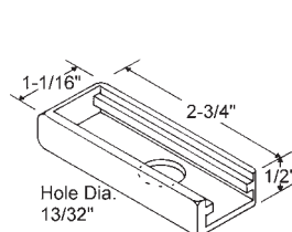
900-20099BE Beige 900-20099B Black 900-20099W White Slide Bolt Cover
