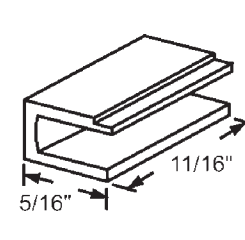
900-6894 Sash Guide
