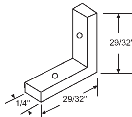
52-603 Slider Corner Angle Die Cast
